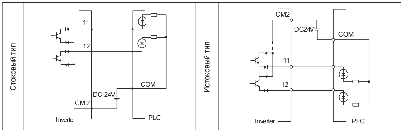
Рис. 2-7 Подключение клемм выхода и программируемого логического контроллера (ПЛК)
