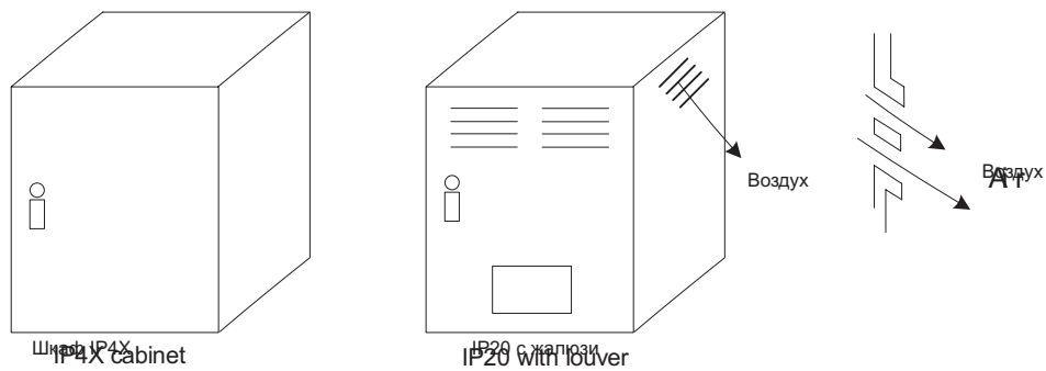
Рис. 1. Шкаф инвертора
