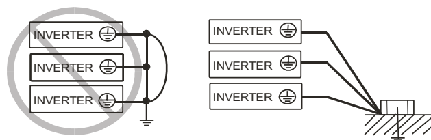
Рис. 2- 4 Заземление (G)
