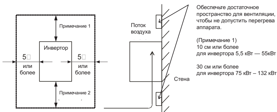
Рис. 2-1 Поверхность для крепления инвертора
