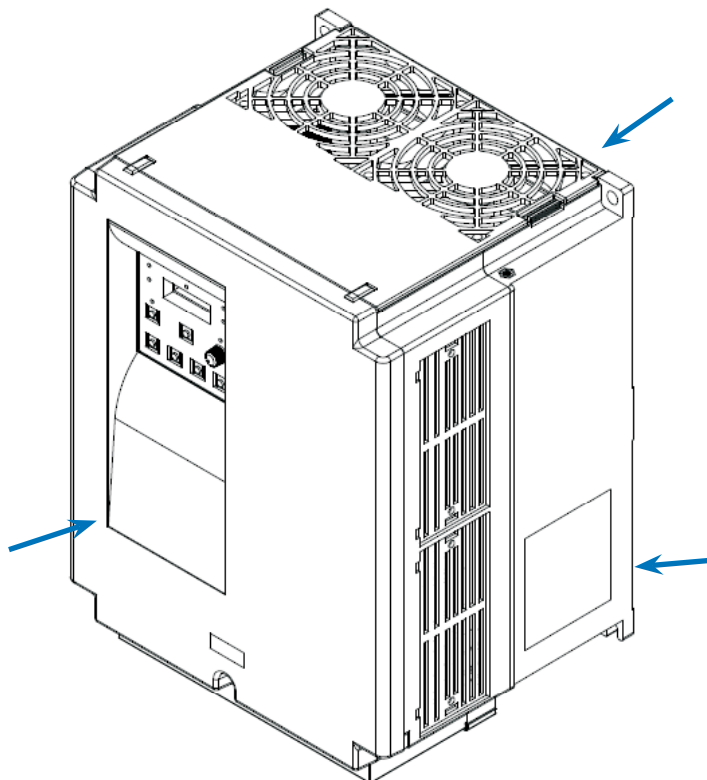
Рис. 2-2 Положение для установки
