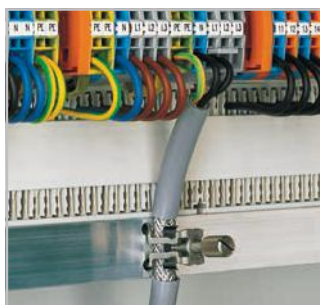
Установка непосредственно на металлическую пластину (максимальная толщина 3 мм)
