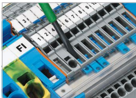
Подключаемый с помощью инструмента N-размыкатель
