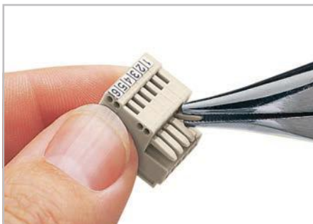
Кодирование розетки – извлечение ключа (-ей) кодировки.
