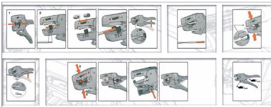
Обрезание проводника.
