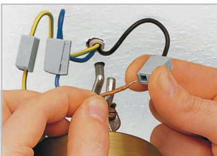
Страна осветительной арматуры: нажмите до упора кнопку, введите в прямоугольное отверстие конец зачищенного проводника и отпустите его.
