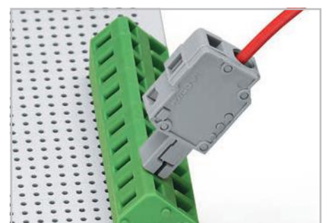
Модуль тестового штекера вставлен, проводники при этом не подключены
