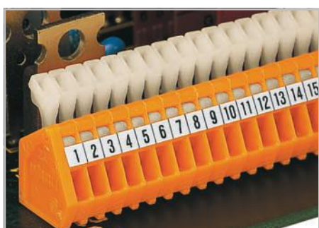
Маркировка с использованием самоклеящихся маркировочных полосок (выше) или прямой заводской маркировки.
