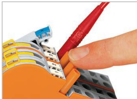
Защищенные от касаний тестовые штекеры 4 мм Ø не поставляются компанией WAGO, но предлагаются такими поставщиками промышленного оборудования, как Fabrikat Multi-Contact.
