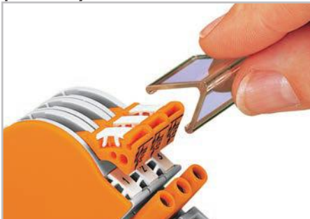
Защелкивающаяся прозрачная крышка на 1 – 8 размыкателей: а) Механическая блокировка нескольких размыкателей для схем коммутации с замыканием нескольких контактов б) Защита маркеров
