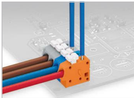
Тестирование при помощи тестового отвода Ø 1 мм – точечный контакт.
