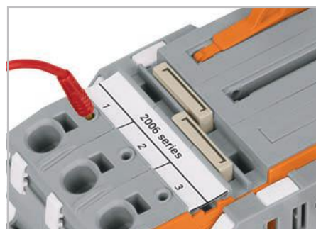
Объединение клемм шириной 15 мм с помощью гребешковых перемычек: от 1 до 3 (2006-433) и от 1 до 5 (2006-435).
